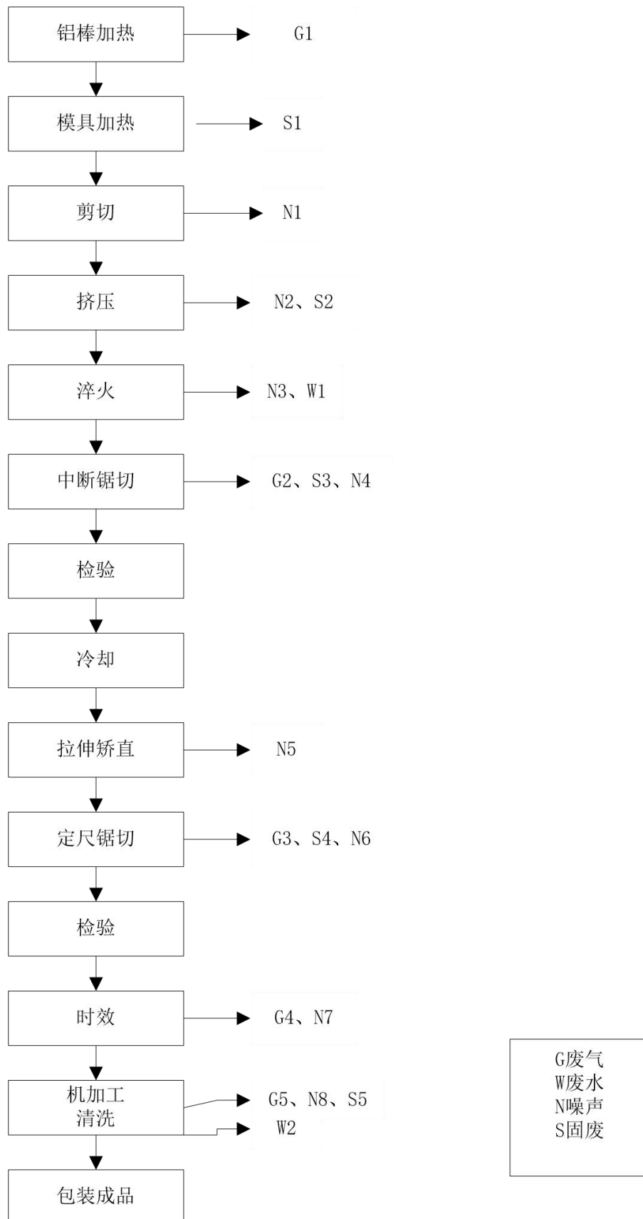
3.4-8 交通运输轻量化铝合金零部件及 IT 配件工艺流程及产物节点图
