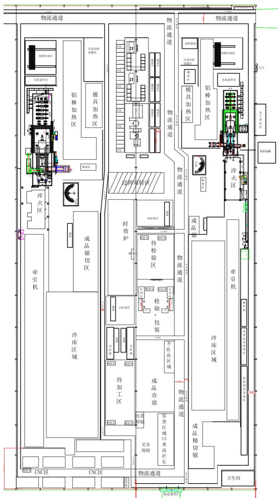
附图 4 年产 2 万吨交通运输轻量化铝合金零部件及 IT 配件项目平面布置图
