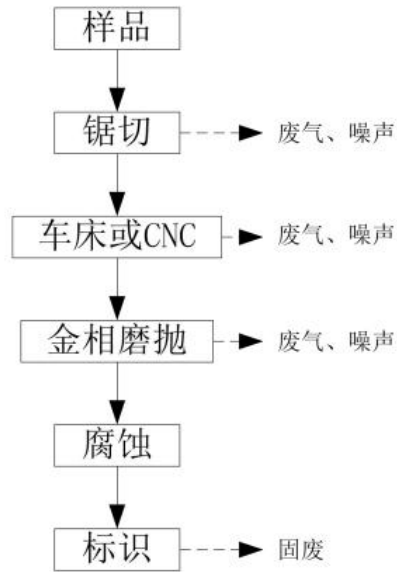
3.4-4 金相样品工艺流程及产物节点图
