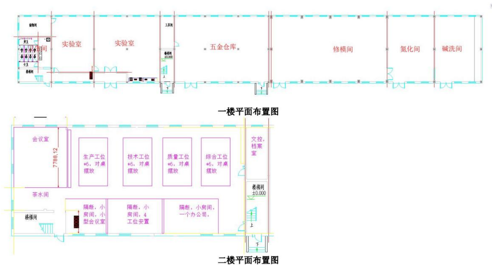
附图3 年产15万吨SMC绿色新型材料综合楼项目平面布置图
