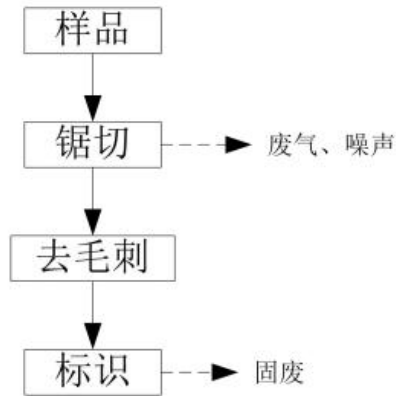
3.4-5 尺寸样品工艺流程及产物节点图
